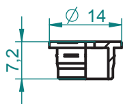
Пробки 3,5 для крышки диаметром 18мм Pourer 3,5 for screwcap 18mm
