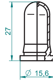
Присоска 1мл Suction cup 1ml
