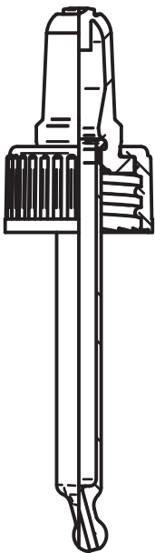
Крышки диаметром 18мм с пипеткой и присоской Screwcap 18mm with pipette and suction cup
