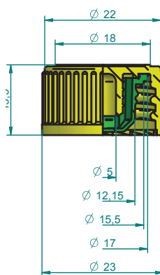
Технический чертёж, пресс-форма Technical project, mould
