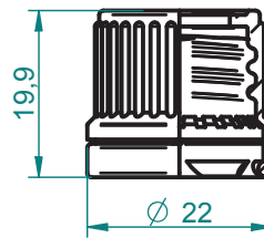
Крышки диаметром 18мм с контрольным кольцом и отверстием для пипетки Screwcap 18mm with tamper evident safety and hole for pipette
