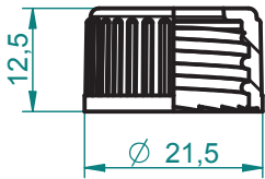
Крышки диаметром 18мм с отверстием для пипетки Screwcap 18mm with hole for pipette
