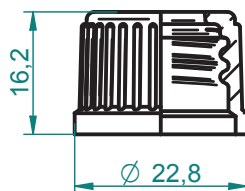
Nakrętka śr.18mm DIN z otworem do pipety Screwcap 18mm DIN with hole for pipette
