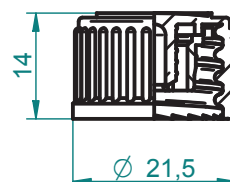
PN*18*OGR*6,0 Nakrętka śr. 18mm z ogranicznikiem wypływu 6,0 Screwcap 18mm with pourer 6,0
