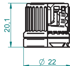
PN*18PII*OGR*6,0 Nakrętka śr. 18mm z pierścieniem gwarancyjnym i ogranicznikiem wypływu 6,0 Screwcap 18mm with tamper evident safety and pourer 6,0
