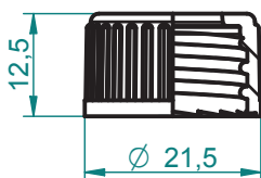
Nakrętka śr.18mm z otworem do pipety Screwcap 18mm with hole for pipette
