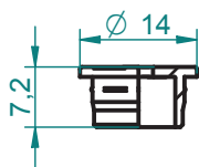
Ogranicznik wypływu 3,5 do nakrętki śr.18mm Pourer 3,5 for screwcap 18mm
