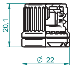
PN*18PII*OGR*3,5 Nakrętka śr. 18mm z pierścieniem gwarancyjnym i ogranicznikiem wypływu 3,5 Screwcap 18mm with tamper evident safety and pourer 3,5
