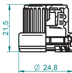
PN*18PIII*OGR*3,5 Nakrętka śr. 18mm z pierścieniem gwarancyjnym typ PIII i ogranicznikiem wypływu 3,5 Screwcap 18mm with tamper evident safety type PIII and pourer 3,5
