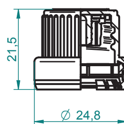
PN*18PIII*OGR*6,0 Nakrętka śr. 18mm z pierścieniem gwarancyjnym typ PIII i ogranicznikiem wypływu 6,0 Screwcap 18mm with tamper evident safety type PIII and pourer 6,0
